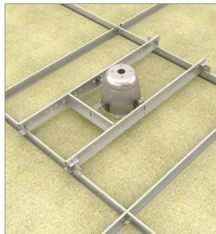
Ovan undertaket används DLC-clips för att fixera avlastningsprofiler vid en belysningsarmatur.
